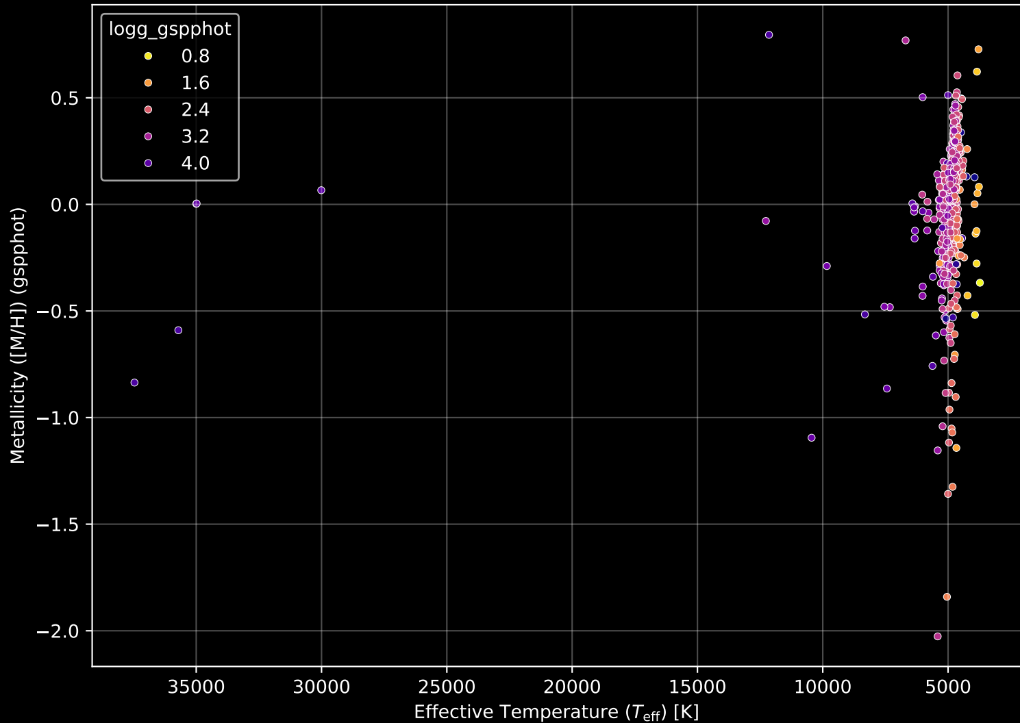
APOGEE DR17 Field: [034+06] Stellar Population Parameters (n= 608)
